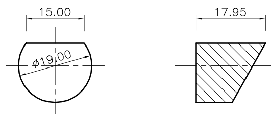
DETALLE DEL TAPON ESCALA 1:1
