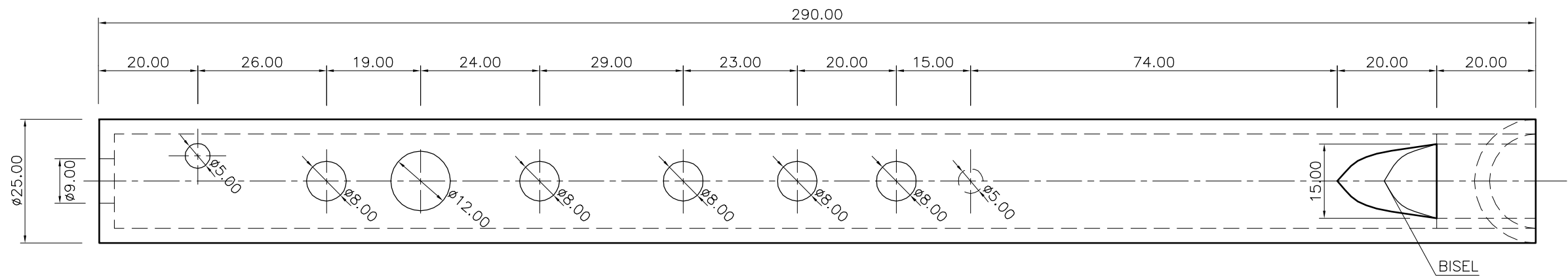
VISTA FRONTAL ESCALA 1:1
