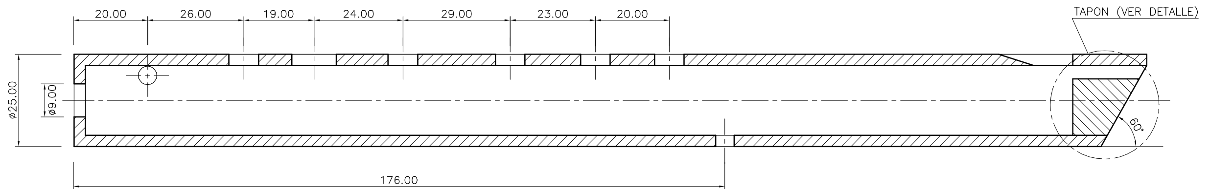
SECCION LONGITUDINAL ESCALA 1:1
